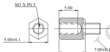
Hex Standoffs SCALE:3/1
